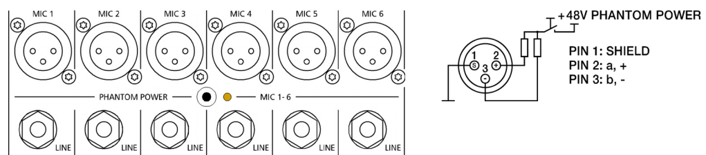
Abbildung 2-1: Mikrofon-Eingänge
