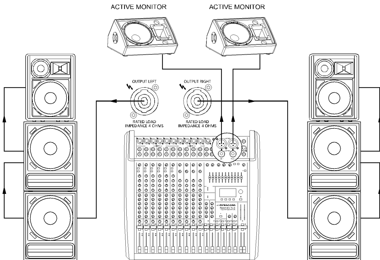
Abbildung 6-1: Maximale Ausbaustufe, Passivbetrieb
