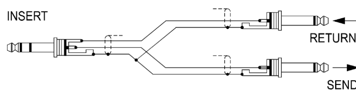
Abbildung 2-3: Y-Kabel für die Verwendung der Insert-Buchse
