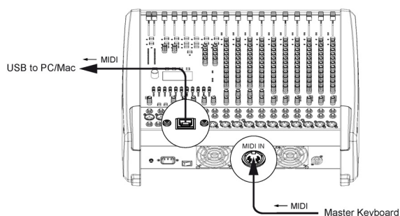
Abbildung 4-5: Übertragung von MIDI-Daten von einem Master Keyboard zum PC/Mac
