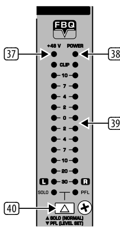
Fig. 2.16: Level meter
