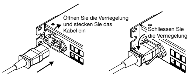
BILD 4:Netzanschluss.
