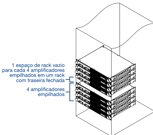
FIG. 2: Como empilhar amplificadores em um rack com a traseira fechada.
