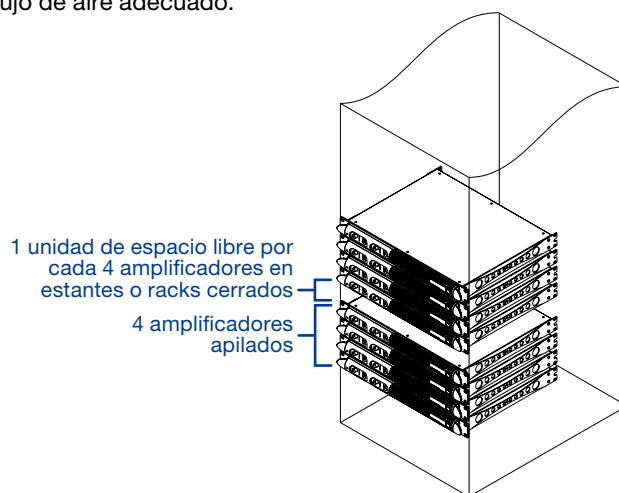
FIG. 2: Como instalar los amplificadores en estantes o racks cerrados.
