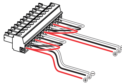
Phoenix MC 1,5/12-ST-3,81 1803675
