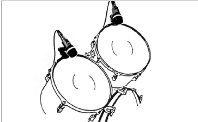
Fig. 5: Orientación del micrófono para tom-tom y roto-tom
