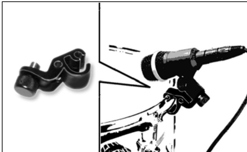
Fig. 4: Sujetar el micrófono en el tom-tom
