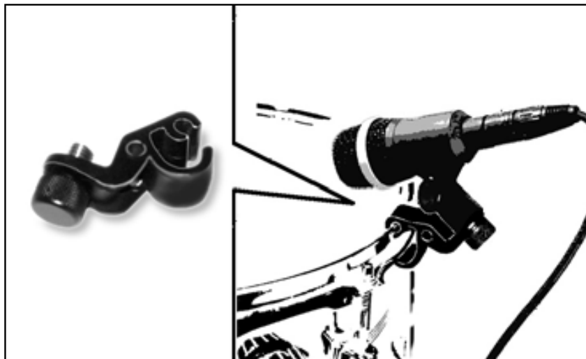
Abb. 4: Mikrofon am Tom-Tom befestigen
